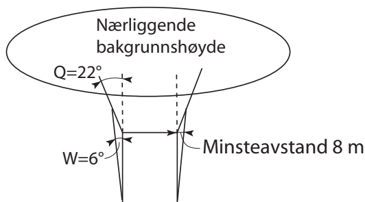
Figur 17A Farlig område i horisontalplanet.
